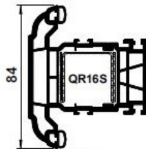
QS16 'T' TRANSOM/ MULLION
