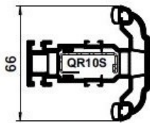
QS10 'T' TRANSOM/ MULLION
